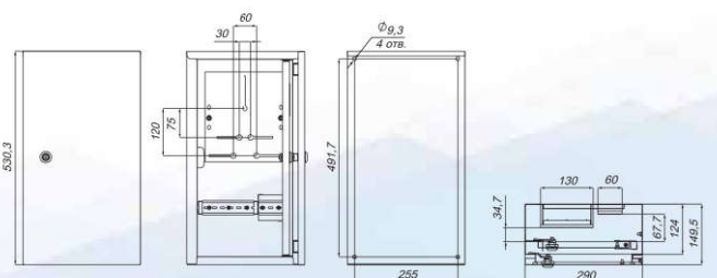
Корпус обліку металевий Light 9 модулів 3фл, навісний IP 54, серії UBox
