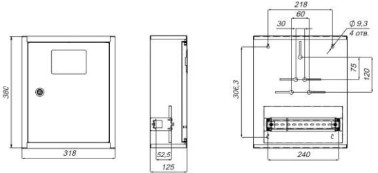
Корпус обліку металевий Light 12 модулів 1фл, навісний IP 31, серії UBox
