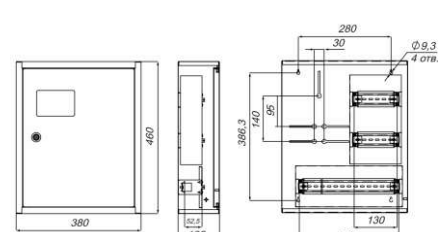
Корпус обліку металевий Light 27 модулів 3фл, навісний IP 31, серії UBox
