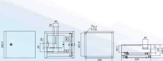
Корпус обліку металевий Light 4 модулі 1фл, навісний IP 54, серії UBox
