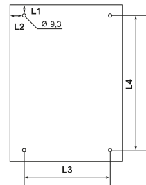
Монтажні отвори навісних корпусів (для всіх типорозмірів)
