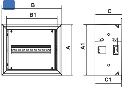
Вбудований корпус (12 модулів)
