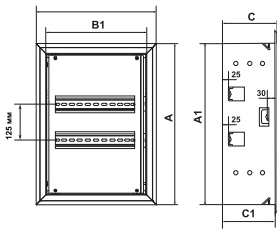
Вбудований корпус (24 модуля)
