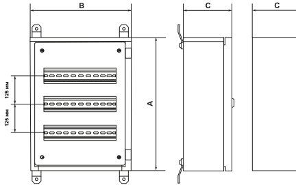
Навісний корпус (36 модулів)
