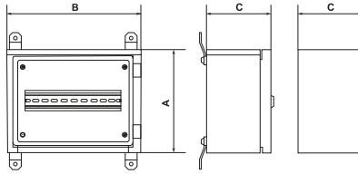
Навісний корпус (12 модулів)
