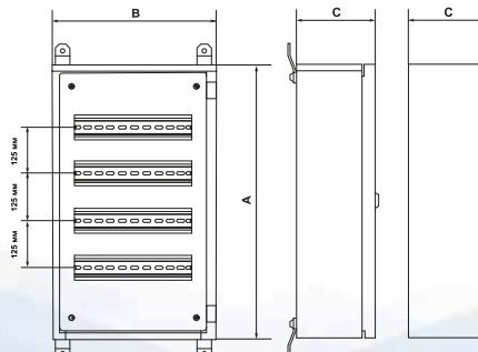
Навісний корпус (48 модулів)
