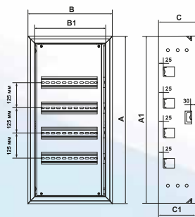
Вбудований корпус (48 модулів)
