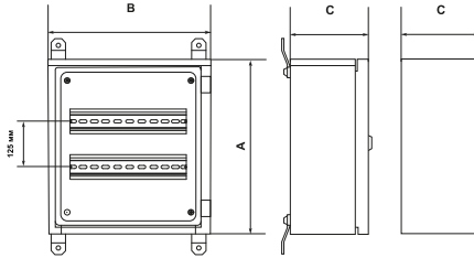
Навісний корпус (24 модуля)
