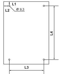
Монтажні отвори навісних корпусів (для всіх типорозмірів)
