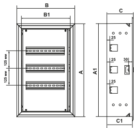
Вбудований корпус (36 модулів)
