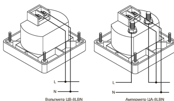
Вольметр ЦВ-8LBN
