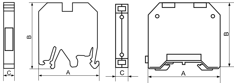
JXB 2,5/35 - 35/35
